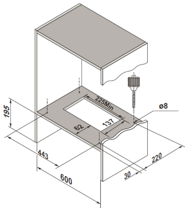
Aktivkohlefilter
