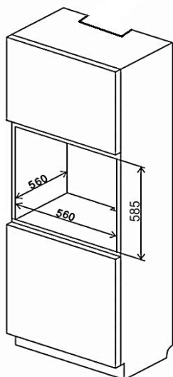
Einbauskitze
