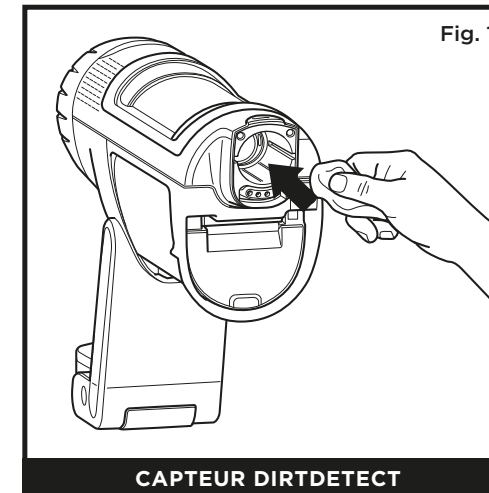
CAPTEUR DIRTDETECT
